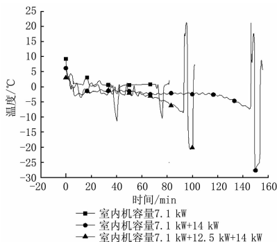
图 3 不同室内机容量吸气温度的变化
