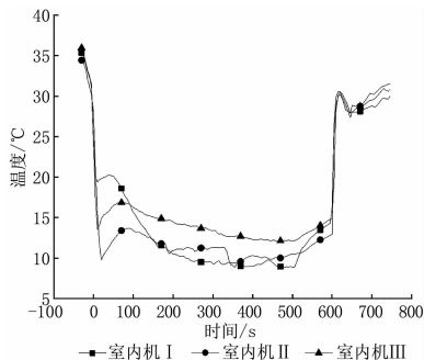
图6 室内机出风温度变化
