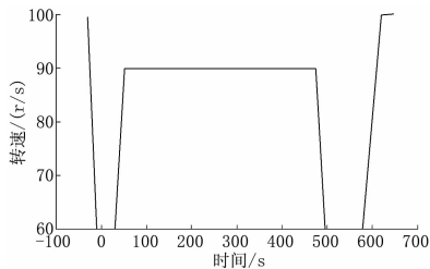
图7 除霜过程中的压缩机转速变化
