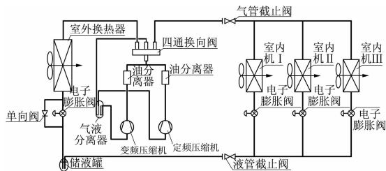
图 2 变频空气源热泵多联机系统原理图
