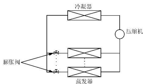
图 1 小型商用集中空调原理图
